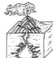
Magma & Lava
